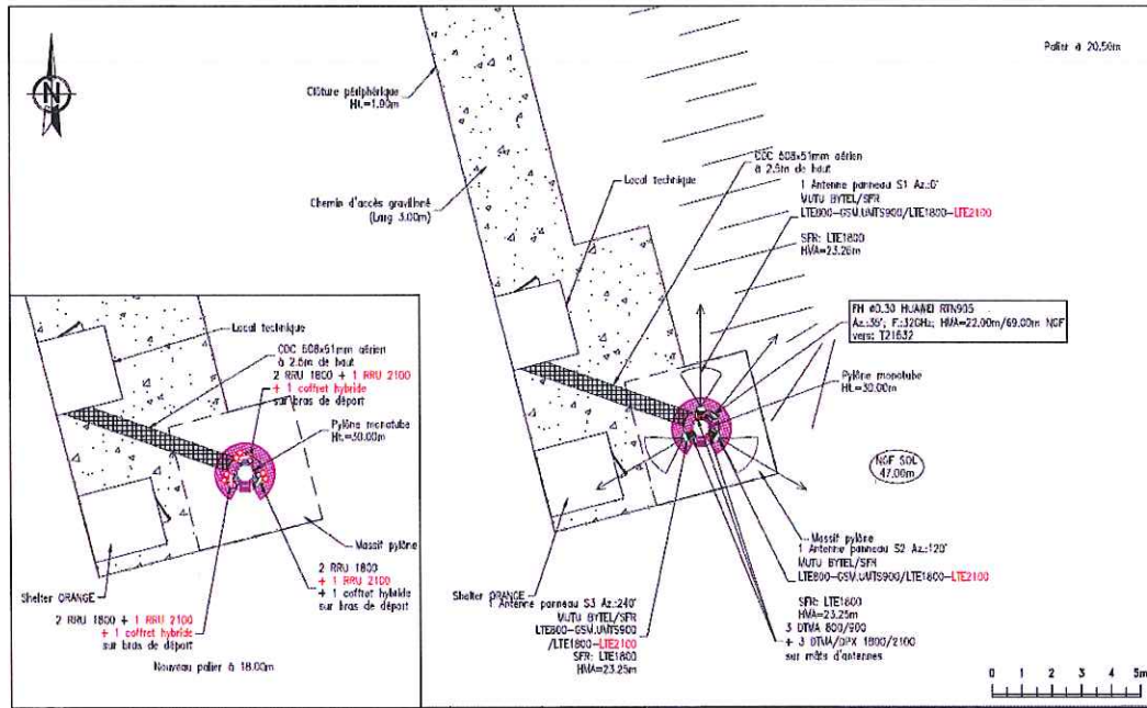
Etat projeté
