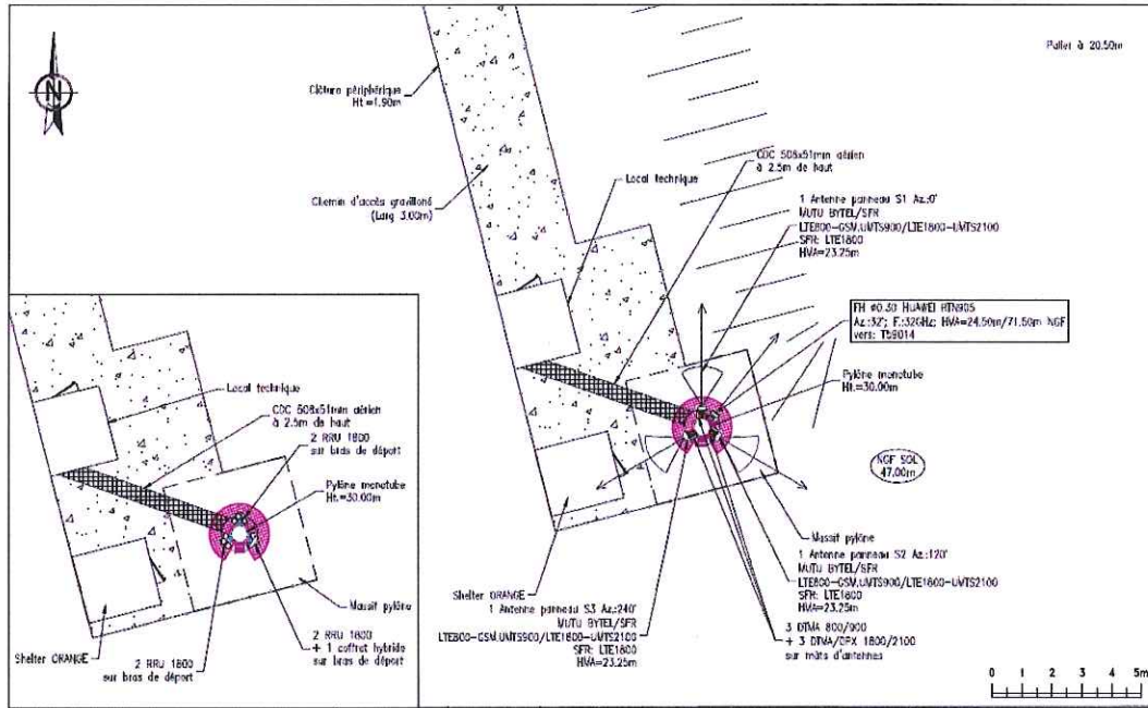
Etat projeté
